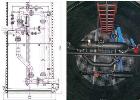
Mess- und Regelschacht DN 2600
